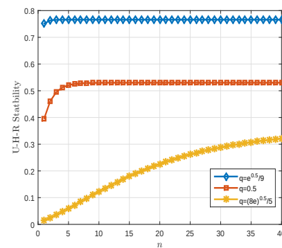
(b) UHR Stability
